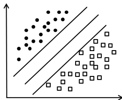
图 1 线性可分下的最优分类
